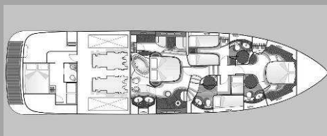
Cubierta inferior
